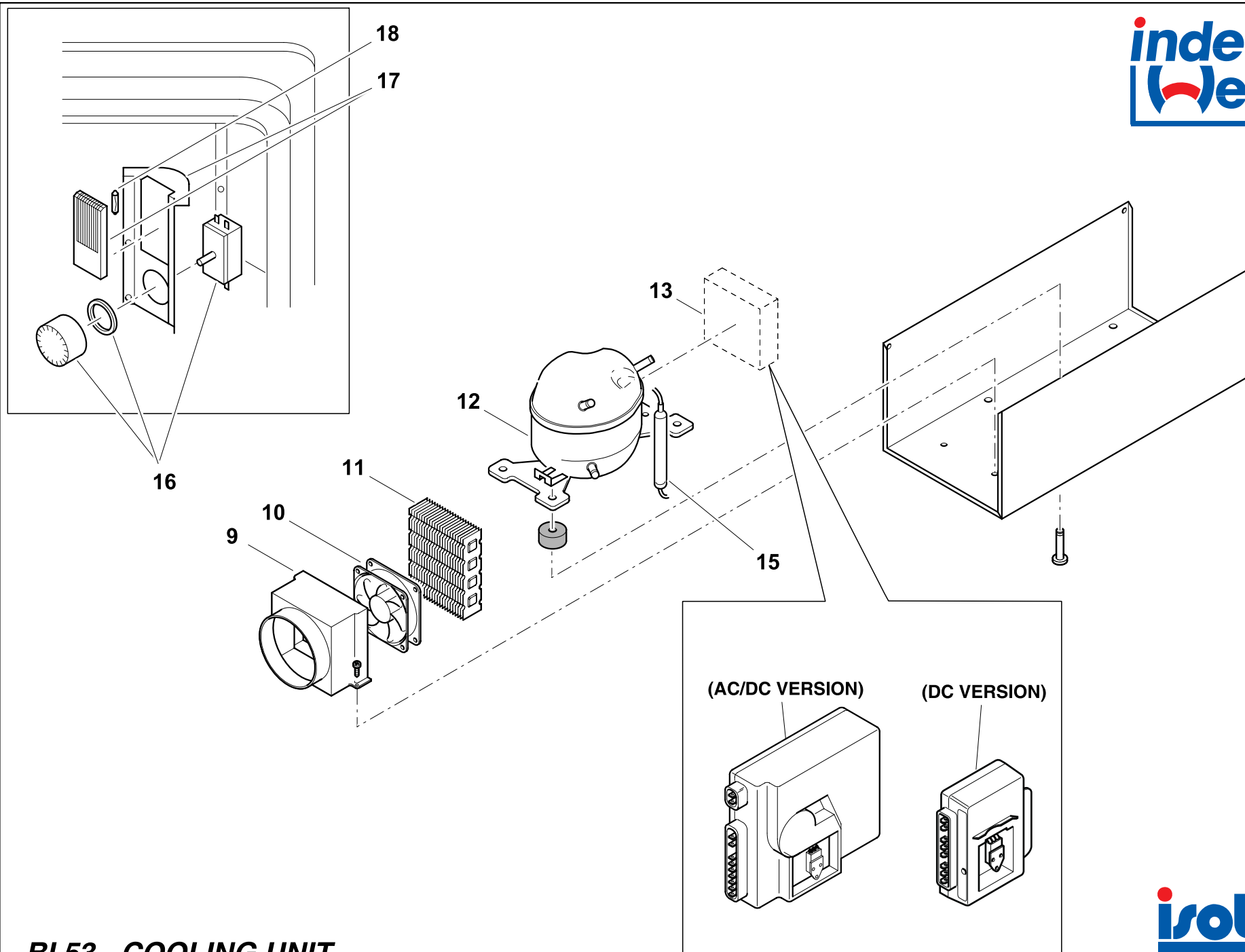
BI 53 - COOLING UNIT
